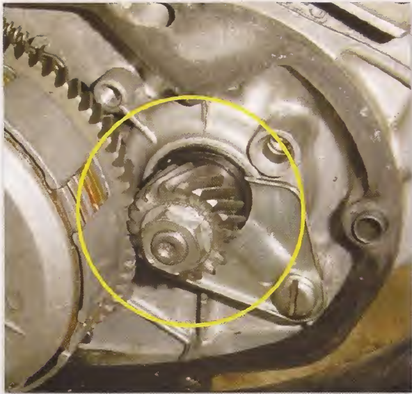
Piñón primario
